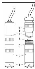
Abb. 3 Trennbarkeit
