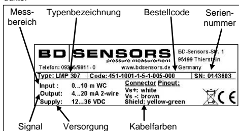
Abb. 1 Typenschild
