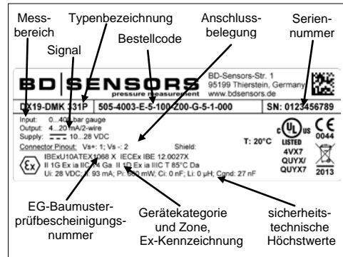
Abb. 1 Typenschild
