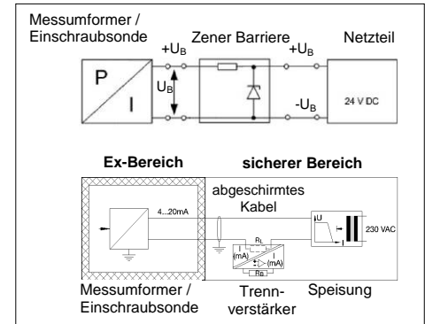
Abb. 3 Schaubilder Beschaltung
